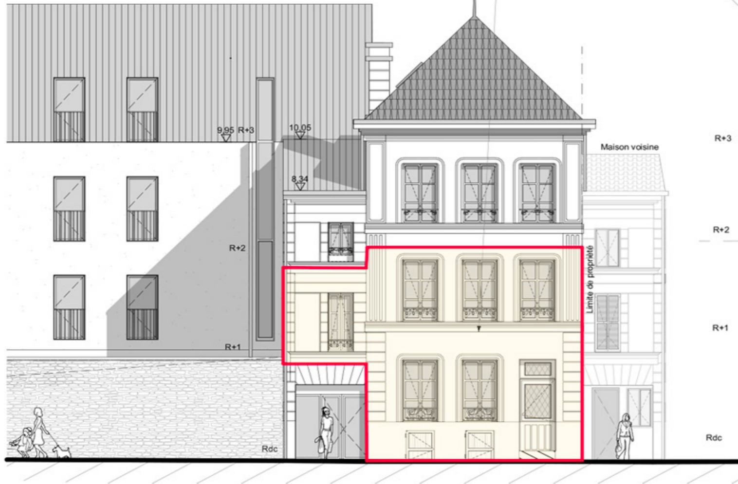
Élévation sur rue Ribray Ech. : 1/200
