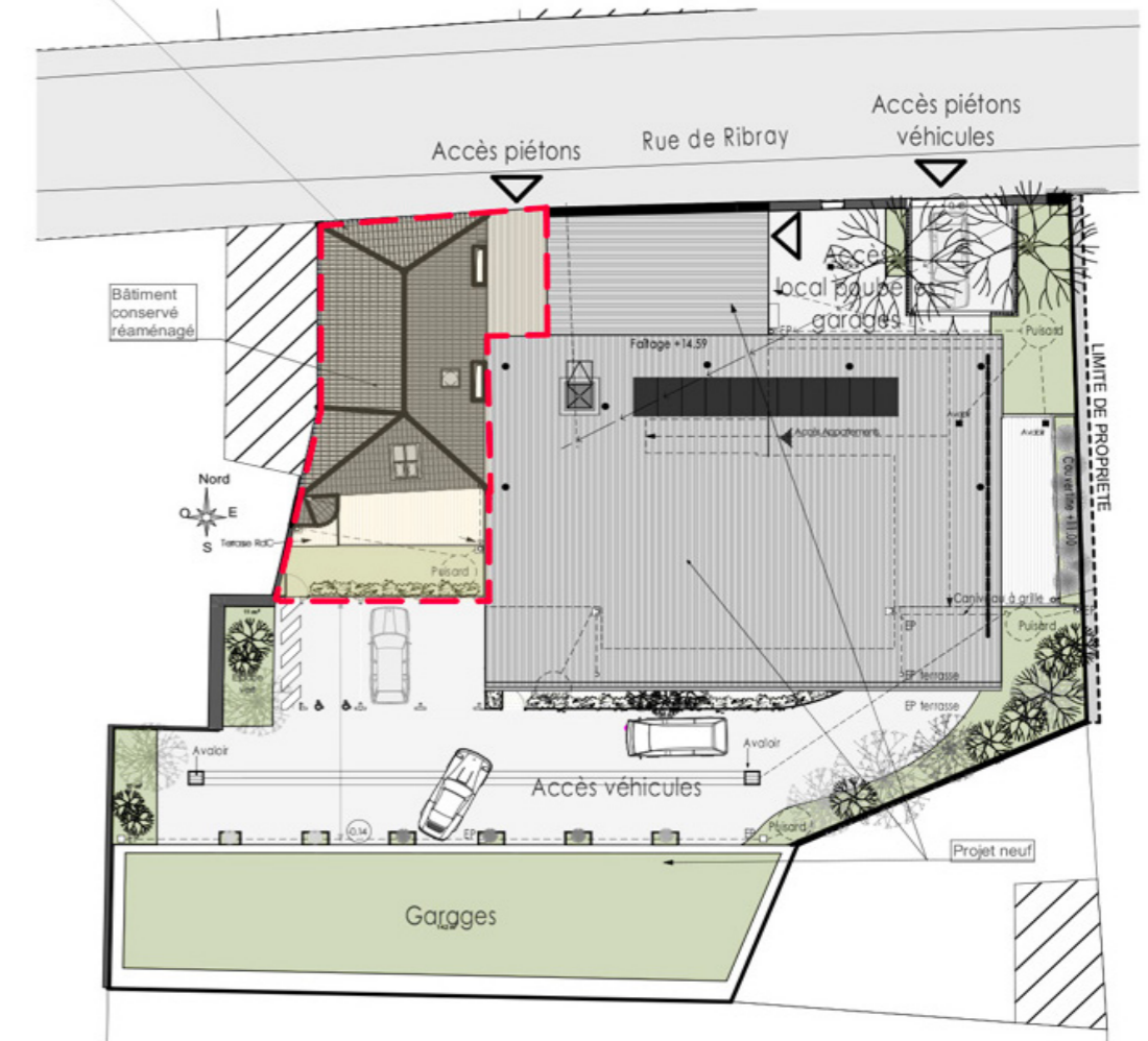
Plan de masse Ech. : 1/500
